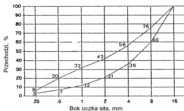
Rysunek 1. Krzywe graniczne uziamienia kruszywa do betonu
