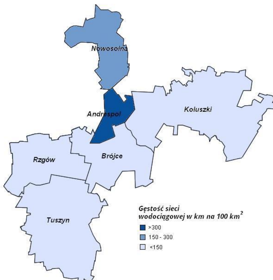
Rysunek 3. Gęstość sieci wodociągowej w Powiecie Łódzkim Wschodnim w podziale na gminy
